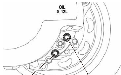
齒輪油放油螺栓
