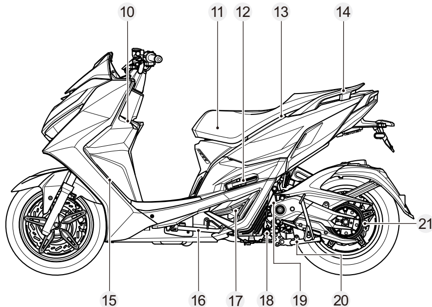
左側視圖 (皮帶版)
