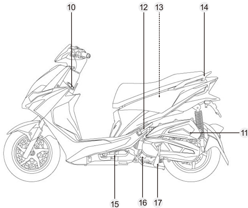
左側視圖
