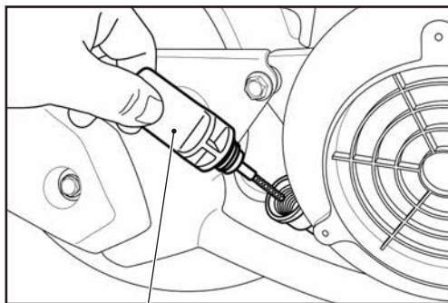
機油量尺
