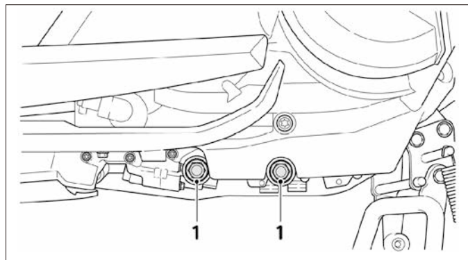
1：洩油螺栓
