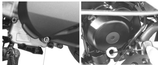
放油螺栓
