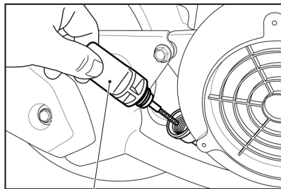
機油量尺
