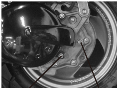
齒輪油放油螺栓
