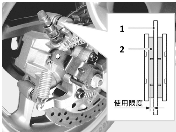
1：煞車碟盤 2：來令片
