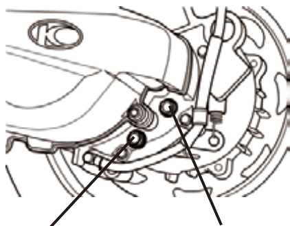
齒輪油放油螺栓
