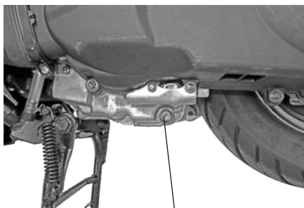
放油螺栓
