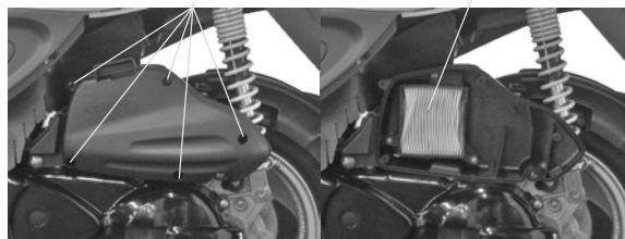
固定螺絲
